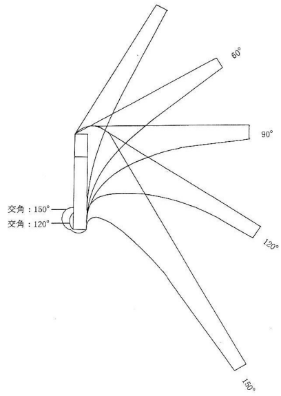
図-1 交差点における車両寸法による分類別軌跡図
