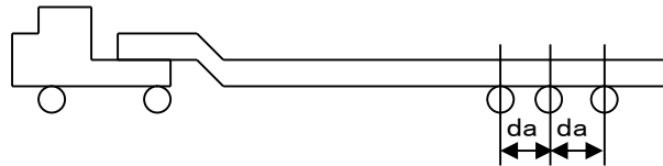
図-3.3 トリプル軸を有する車両
